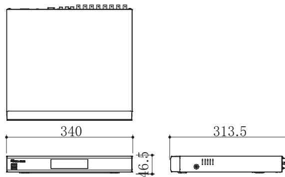
寸法図
