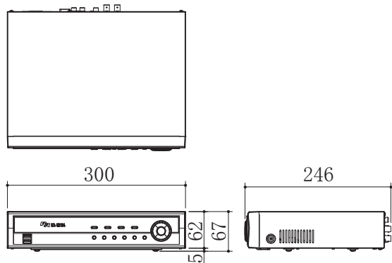
寸法図
